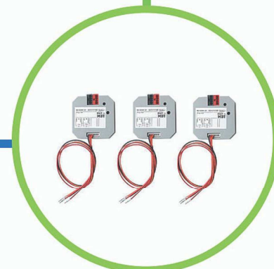
Interfaccia tasti KNX per pulsantiere tradizionali
